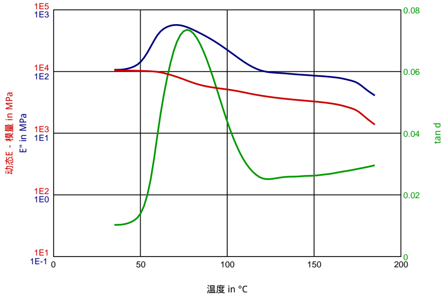
动态E - 模量 - 温度 (干)(measured on Zytel® 70G35HSLR BK099)
